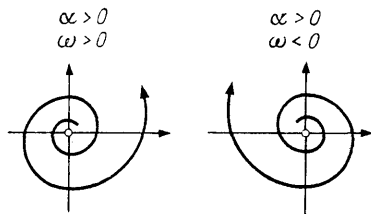
Fig. 124. Unstable foci
