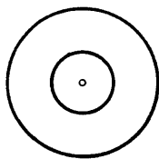
Fig. 125. A center
