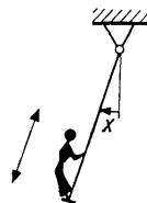
Fig. 192. A swing
