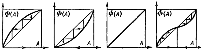
Fig. 18. Lamerey diagrams
